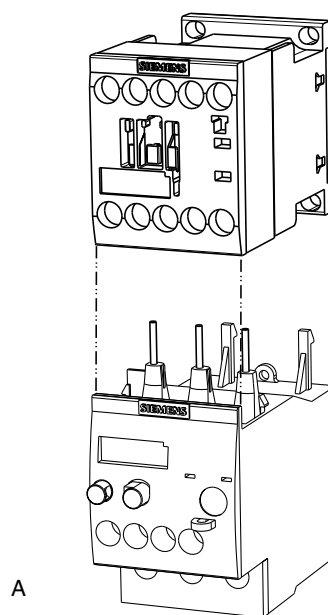
Figuur 7: Motorbeveiligingsschakelaar DOL
