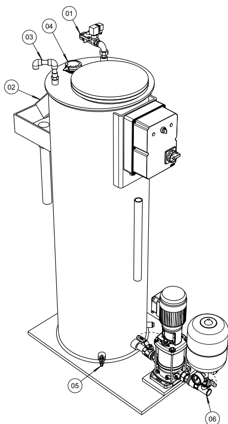
Figuur 2: Installaties van het type Break-Unit AB-onderbreking
