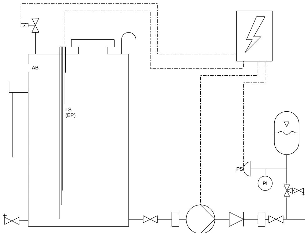
Figuur 8: PI&D Schema HUV1 PW met AB overstort
