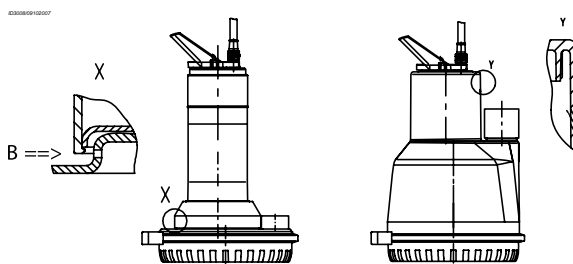
Figuur 2: ontluchtingsgaatje DVV7(K) en DVV10
