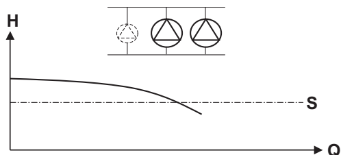
Figuur 10: 2 Hoofdpompen
