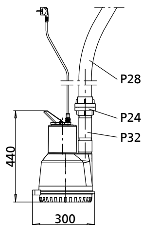
Afb. 13: Maattekening DVV 7 W K
