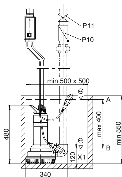
Afb. 11: Maattekening DVV 1022
