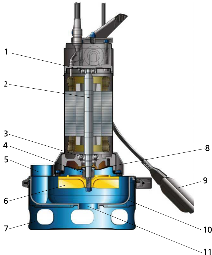
Afb. 2: Doorsnedetekening
