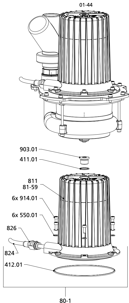
Afb. 38: Explosietekening C1 S 315 40 I - roterend gedeelte
