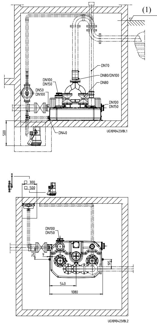
Afb. 45: Aansluitvoorbeeld Feka-Unit C2 V 67, C2 S 315 150 I
