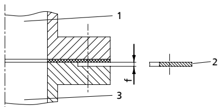
Afb. 8: Flensverbinding
