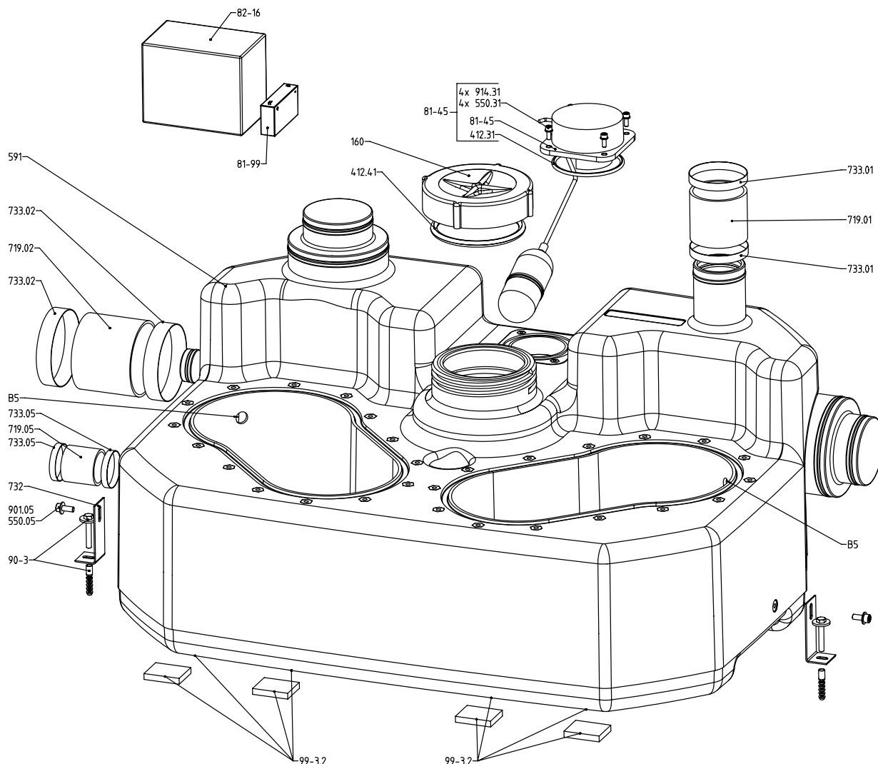
Afb. 43: Explosietekening Feka-Unit C2 S 315 150 I - verzamelreservoir
