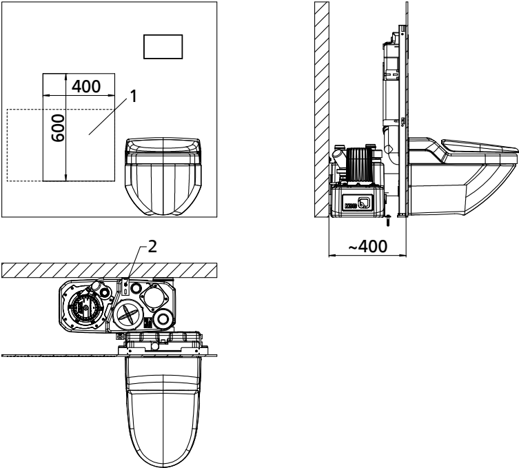
Afb. 46: Achterwandmontage
