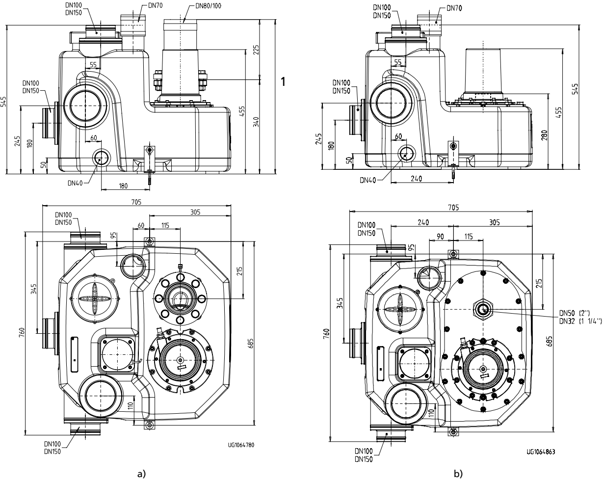
Afb. 48: Maten Feka-Unit a) C1 V 915 en b) C1 S 315 100 I Maten in [mm]
