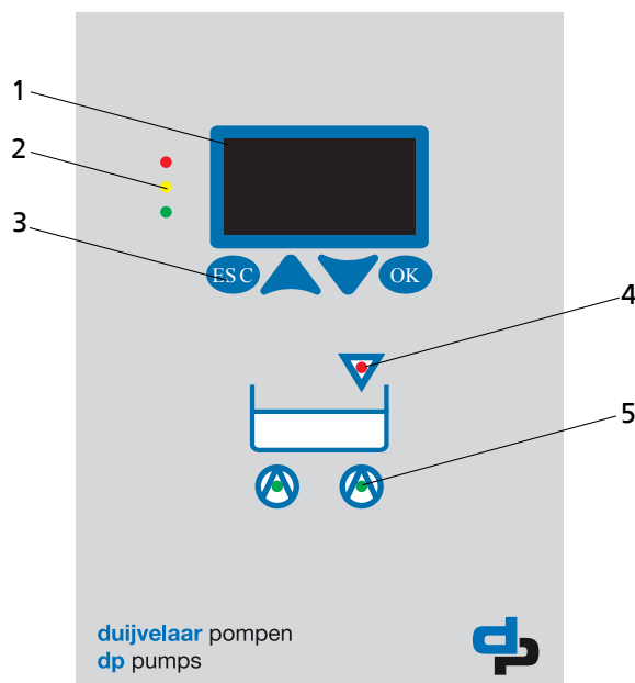
Afb. 18: Bedieningspaneel
