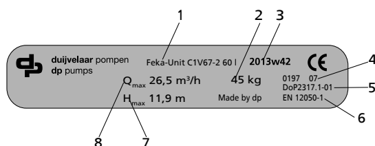
Afb. 2: Typeplaatje (voorbeeld)
