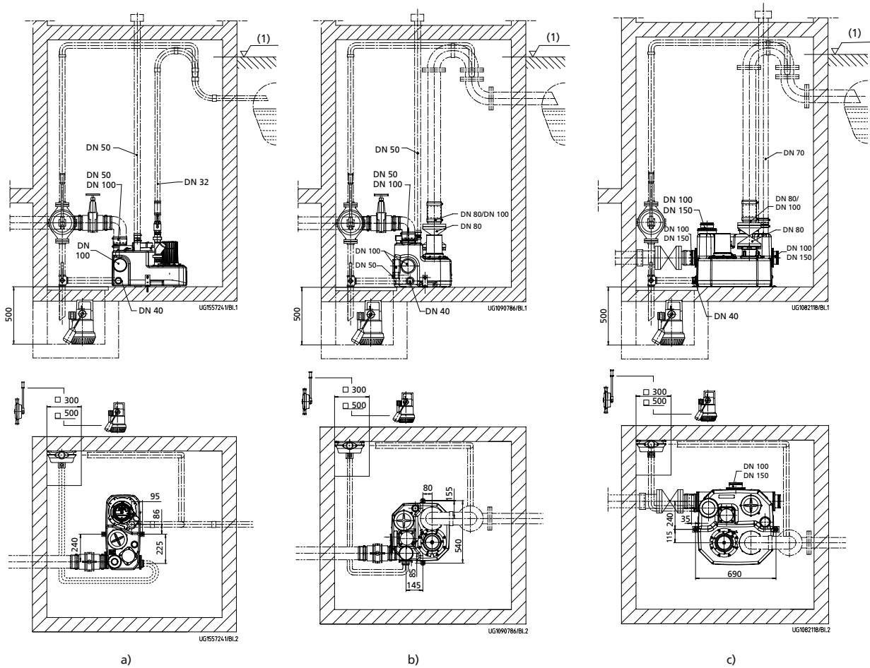
Afb. 44: Aansluitvoorbeeld Feka-Unit
