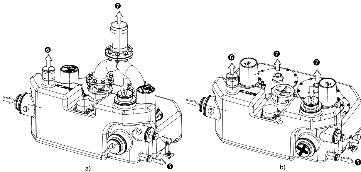
Afb. 56: Aansluitingen mini-Compacta a) UZ150 b) UZS150
