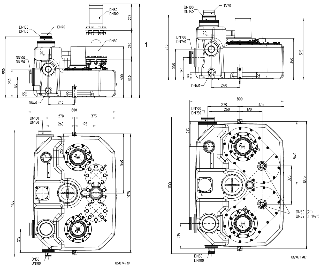
a) b) Afb. 49: Maten Feka-Unit a) C2 V 67 150 I en b) C2 S 315 150 I Maten in [mm]
