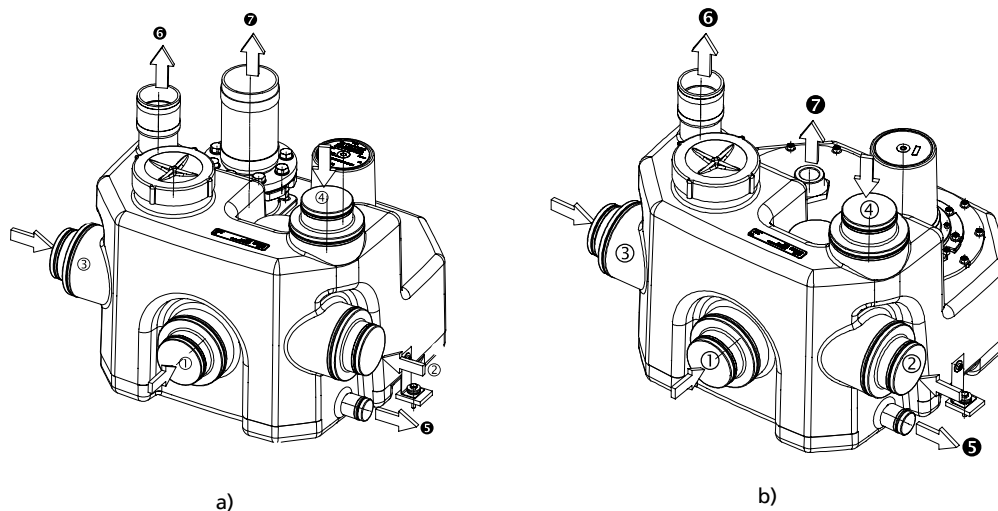
Afb. 55: Aansluitingen Feka-Unit a) C1 V 915 en b) C1 S 315-2 100 I
