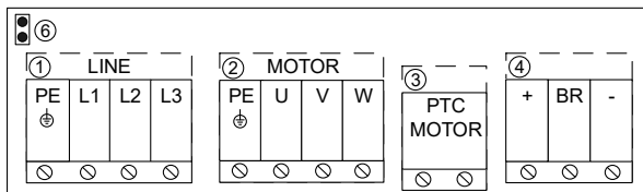
Afb. 11: Overzicht klemmenstrips bij uitvoering 400 V/ 3~ met 2 relais
