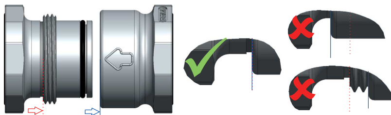
Afb. 40: Uitlijning controleren
