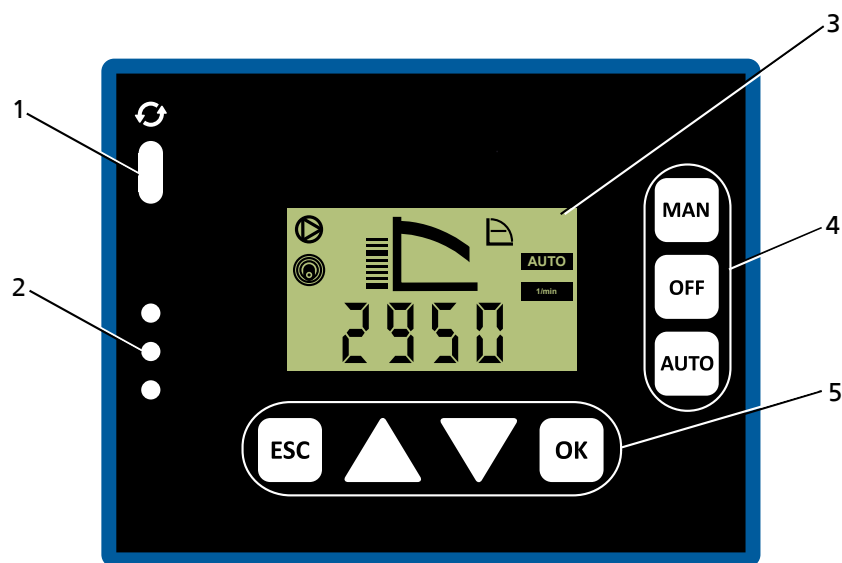
Afb. 30: Standaard bedieningspaneel
