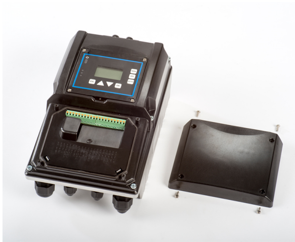
Afb. 12: Huisafdichting
