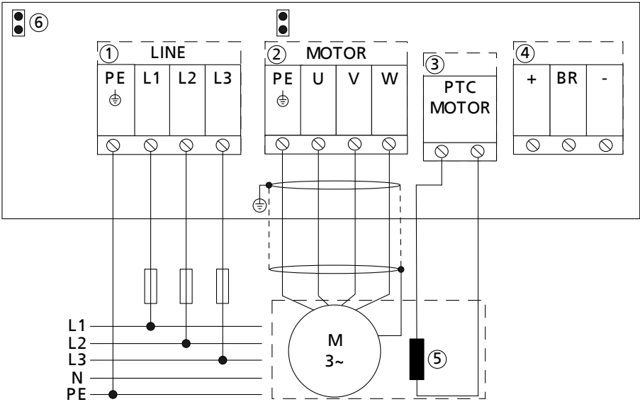
Afb. 18: Stroomnet- en motoraansluiting aansluiten grootte B
