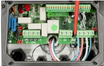
Afb. 27: Motorkabels aansluiten
