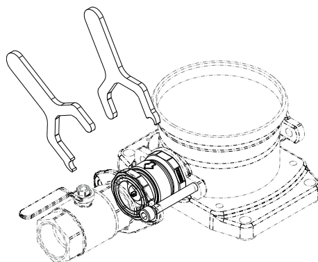
Afb. 36: Delen van de behuizing in elkaar schroeven
